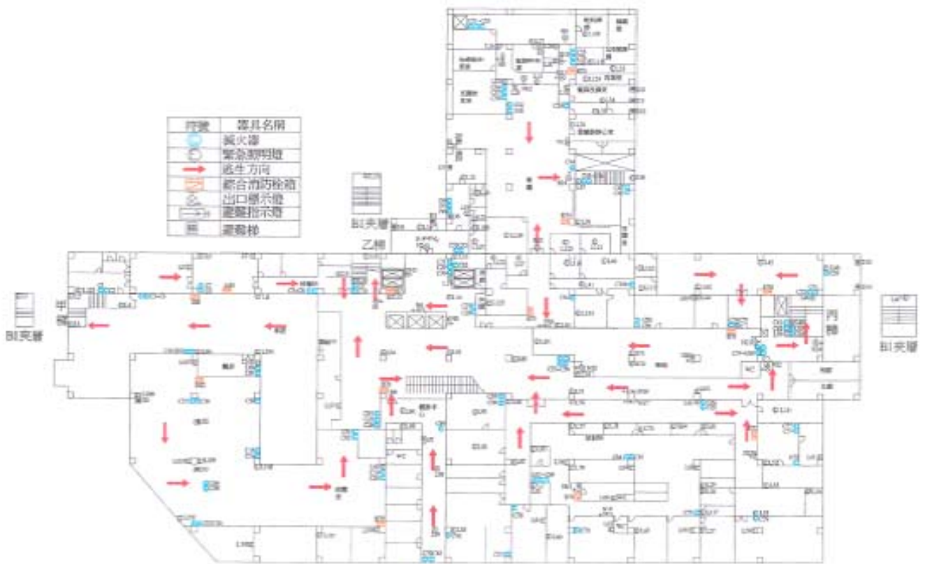
第一醫療大樓地下一樓逃生路線圖
