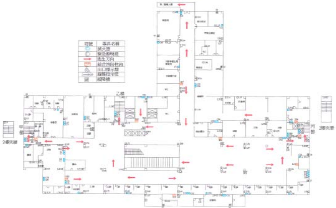
第一醫療大樓二樓逃生路線圖
