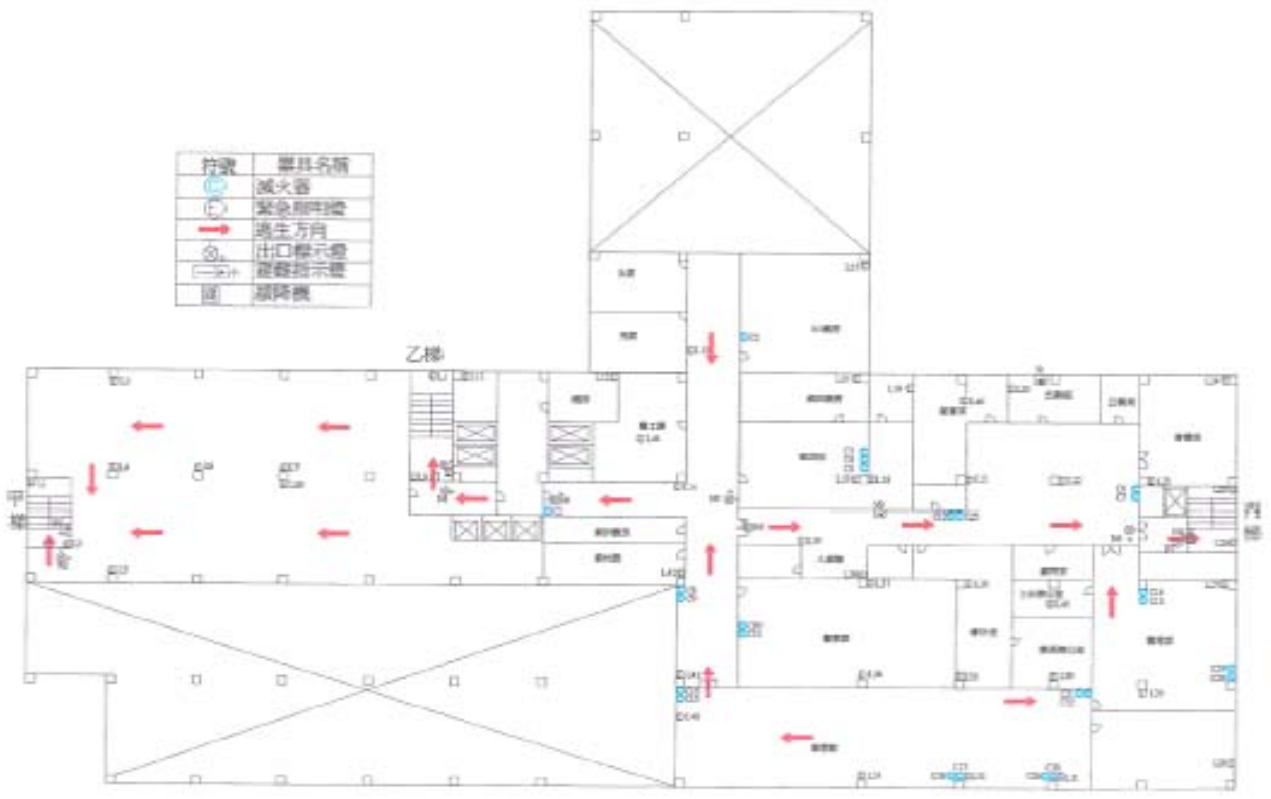
第一醫療大樓3A逃生路線圖
