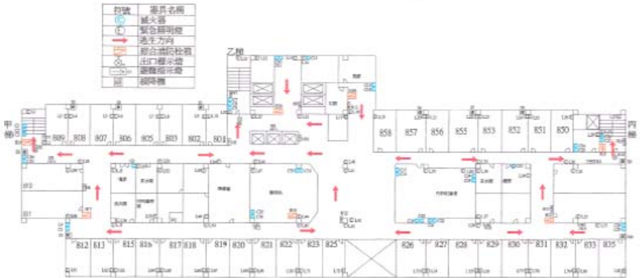
第一醫療大樓八樓逃生路線圖
